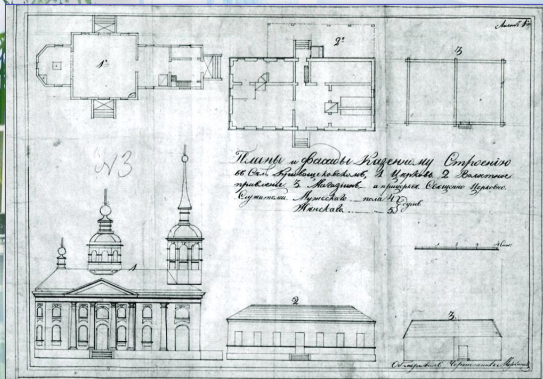
План Никольской церкви с. Кривошеиково
